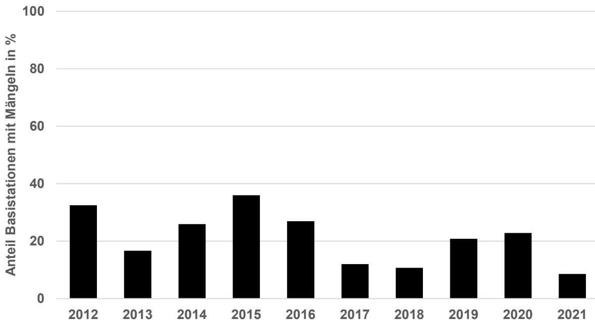
Abbildung 2: Anteil kontrollierter Basisstationen mit mindestens einem Mangel
