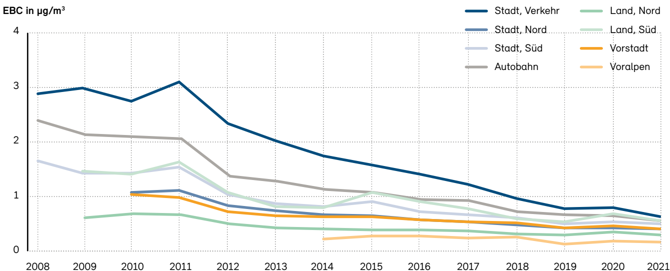
Abb. 11: Jahresmittel von Russ (EBC = equivalent black carbon)
