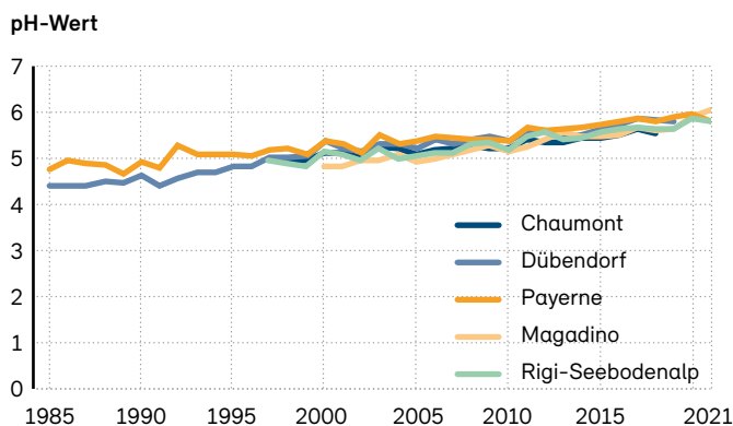
Abb. 17: Säuregehalt von Niederschlag (pH-Wert)
