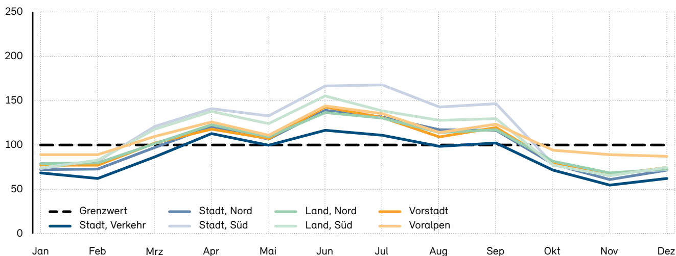
Abb. 14: Monatliche 98-Perzentilwerte der Halbstundenmittel von Ozon im Jahr 2021
