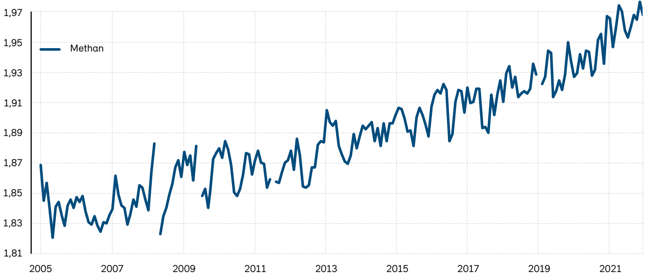
Abb. 24: Monatsmittel von Methan auf dem Jungfraujoch
