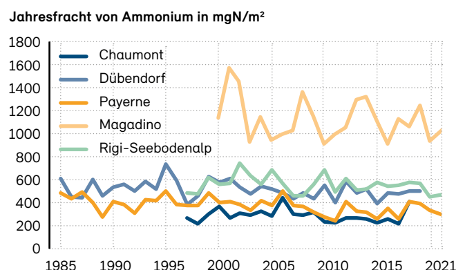
Abb. 20: Jahresfracht von Ammonium im Niederschlag
