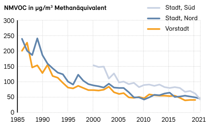
Abb. 22: Jahresmittel von flüchtigen organischen Verbindungen ohne Methan (NMVOC)
