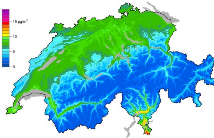
Abb. 3: Karte der Jahresmittel von Feinstaub (PM2.5) für das Jahr 2021 (Grenzwert 10 \mu\text{g}/\text{m}^3 )
