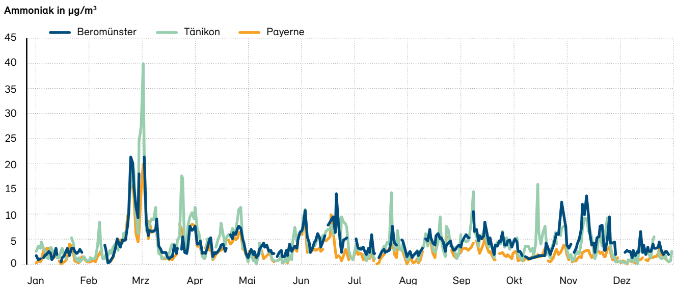
Abb. 16: Tagesmittel von Ammoniak im Jahr 2021
