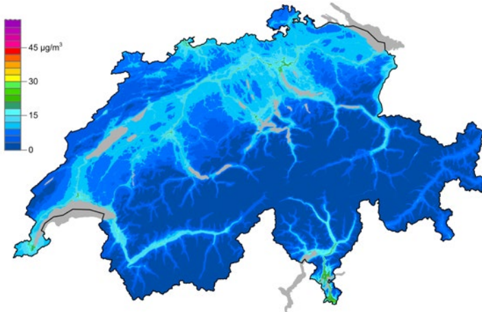
Abb. 2: Karte der Jahresmittel von Stickstoffdioxid für das Jahr 2021 (Grenzwert 30 \mu\text{g}/\text{m}^3 )
