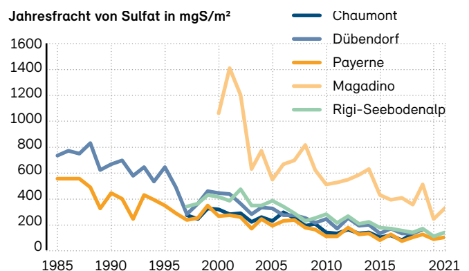
Abb. 18: Jahresfracht von Sulfat im Niederschlag
