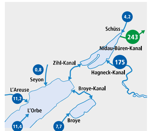
Langjährige Mittel (in m 3 /s) der Zuflüsse in die drei Jurarandseen und des Aare-Abflusses im Nidau-Büren-Kanal.
