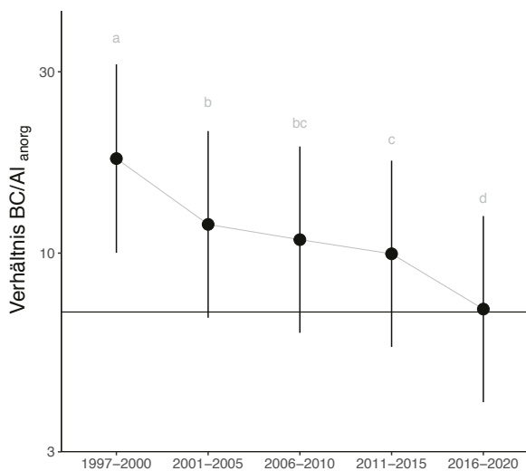
Trend in der Bodenlösung 1997–2020, gemessen in 20–80 cm Tiefe an 47 Standorten der interkantonalen Walddauerbeobachtung, verteilt über die gesamte Schweiz. Das BC/Al-Verhältnis (das Verhältnis der basischen Kationen Kalzium, Magnesium und Kalium zu Aluminium) ist ein wichtiger Indikator für die Bodenversauerung: je tiefer der Wert, desto saurer der Boden. Linie: kritische Grenze von BC/Al = 7 IAP 2021
