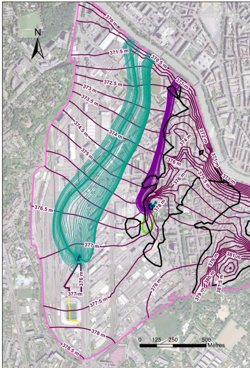
Figure 18 : Ecoulement dans le magasin aquifère de la Praille. On distingue les lignes équipotentiellles (équadistance 0.5 m, en violet) qui constituent la carte piézométrique, les lignes de courants issues des puits de réinjection de la station TAMOIL au Nord du centre commercial de la Praille et les lignes de courant de la réinjection issue des eaux récupérées par le centre commercial MIGROS. La ligne de pression nulle, correspondant à la surface libre de l'aquifère est également représentée (en noir)
