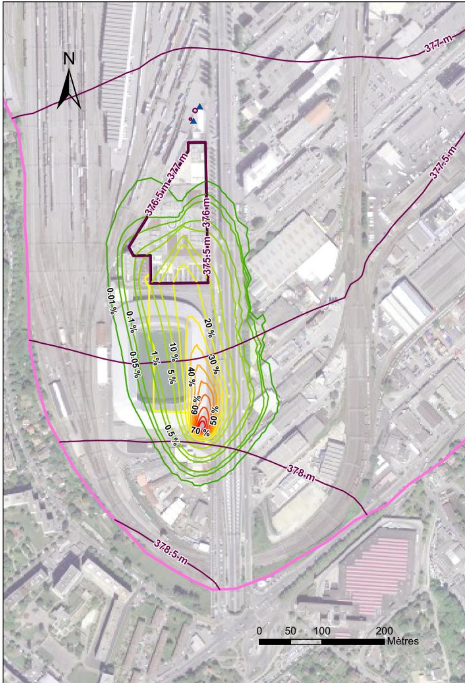
Figure 19 : Panache de contamination issu d'une charge (flux massique) unitaire située juste à l'aval hydraulique immédiat de l'ancien site du CIDEC
