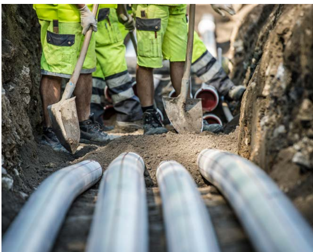
Utilisation de REB® – Ragazer Erdbeton à Coire
