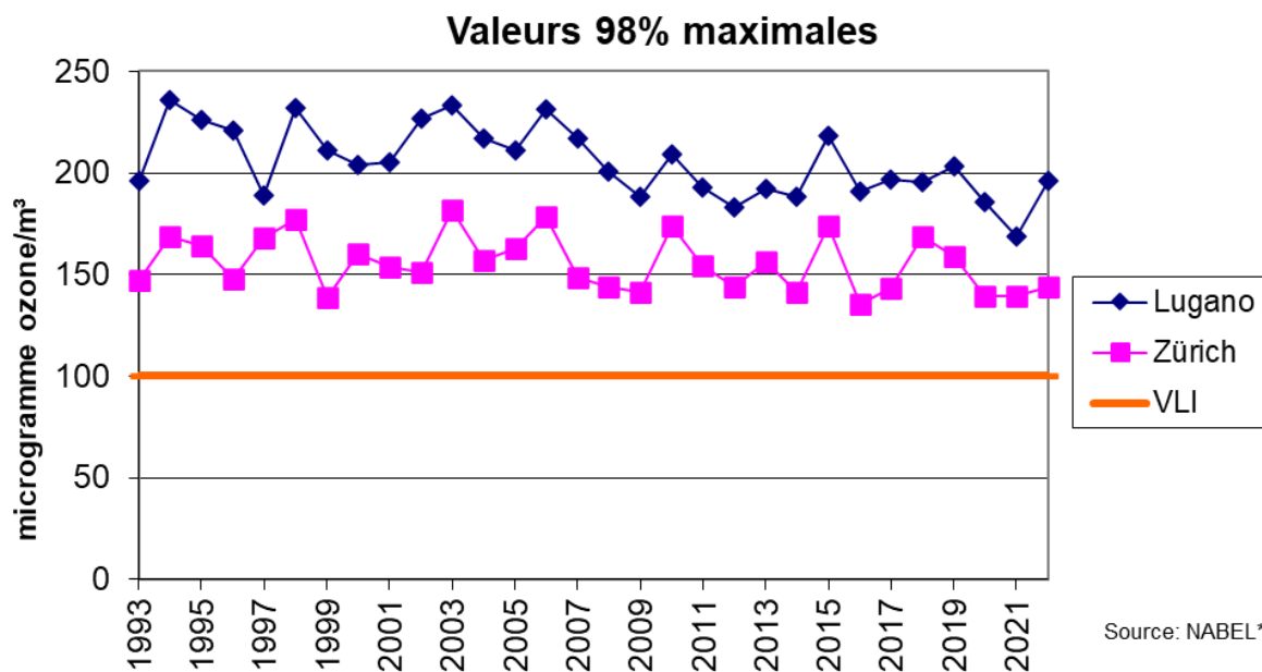
Fig. 1 : Charge en ozone décrite par la moyenne mensuelle la plus élevée de 98% des valeurs semi-horaires
