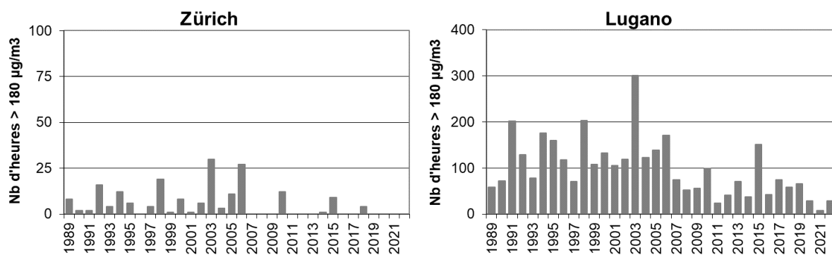
Fig. 3 : Nombre d'heures de dépassements de la valeur de 180 µg/m 3 à Zürich et à Lugano entre 1989 et 2022 (source : NABEL)
