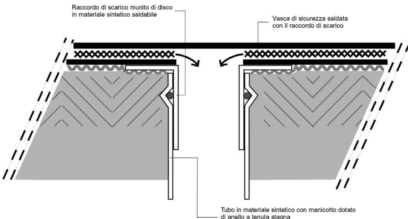
Fig. 18: Dettaglio del sistema di rilevamento delle perdite (esempio)
