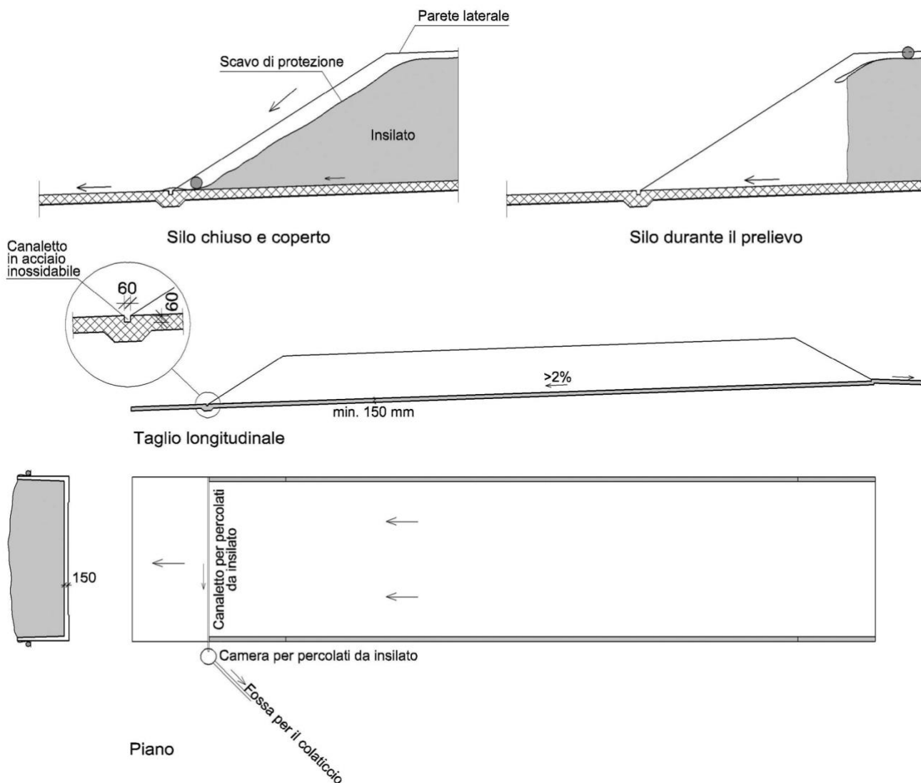
Fig. 11: Esempio schematico di un silo a trincea con canaletto per i percolati da insilato in acciaio inossidabile (dimensioni in mm)
