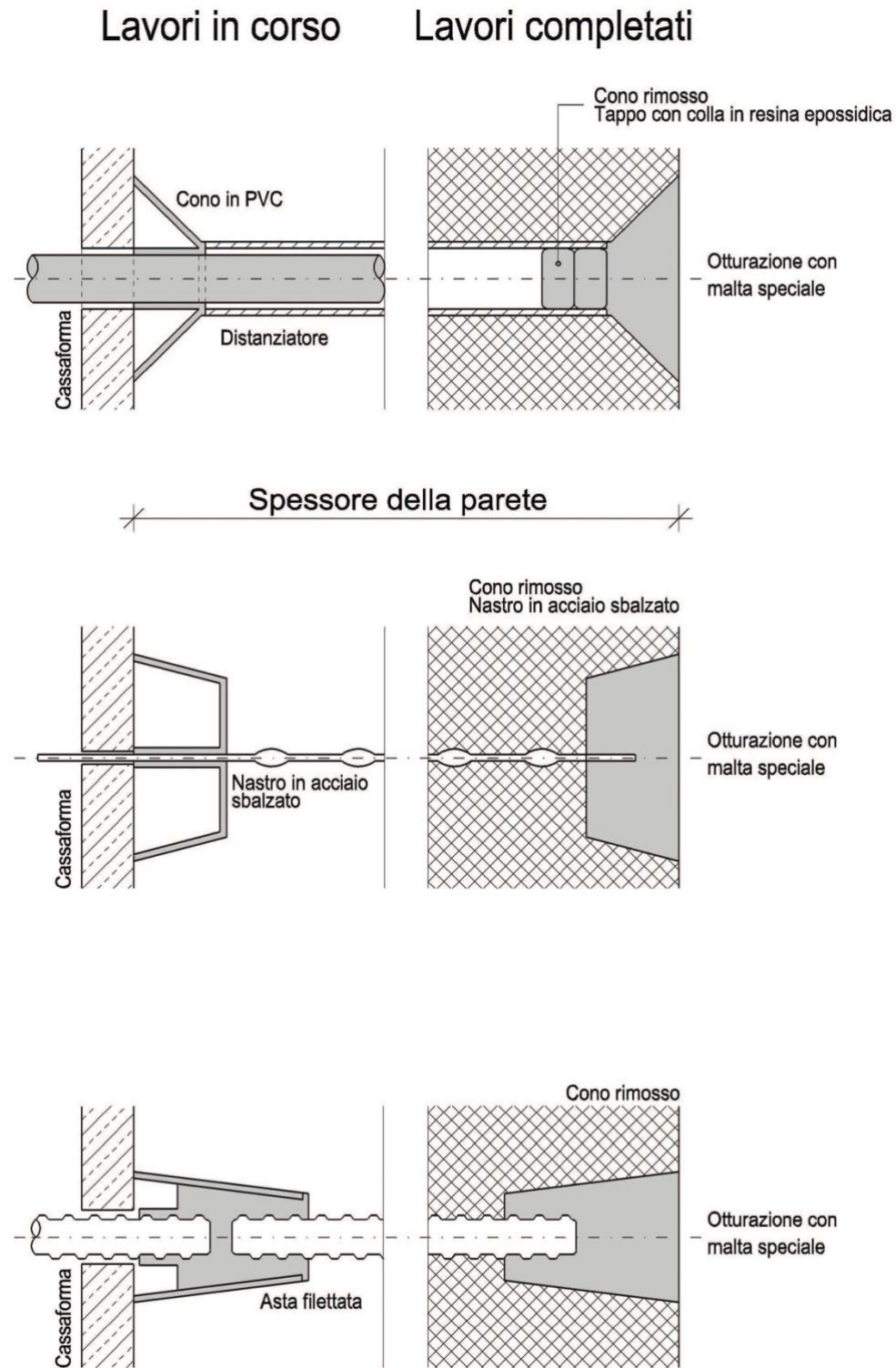
Fig. 5: Esempio di sistemi di assemblaggio per pareti in calcestruzzo a tenuta stagna
