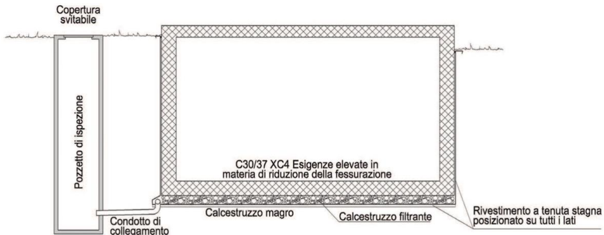
Fig. 13: Esempio di serbatoio del colaticcio con sistema di rilevamento di perdite con rivestimento continuo a tenuta stagna
