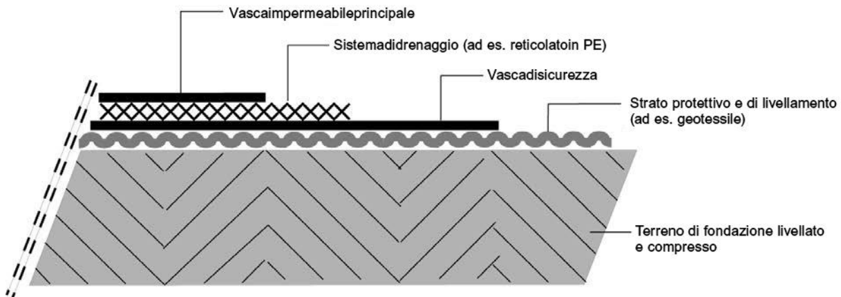
Fig. 16: Caratteristiche del fondo delle vasche (esempio)
