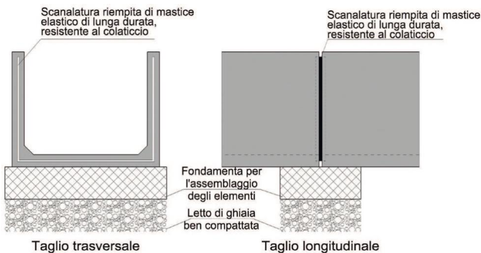
Fig. 9: Canali di smaltimento e canali di raccolta del colaticcio in elementi di calcestruzzo prefabbricati
