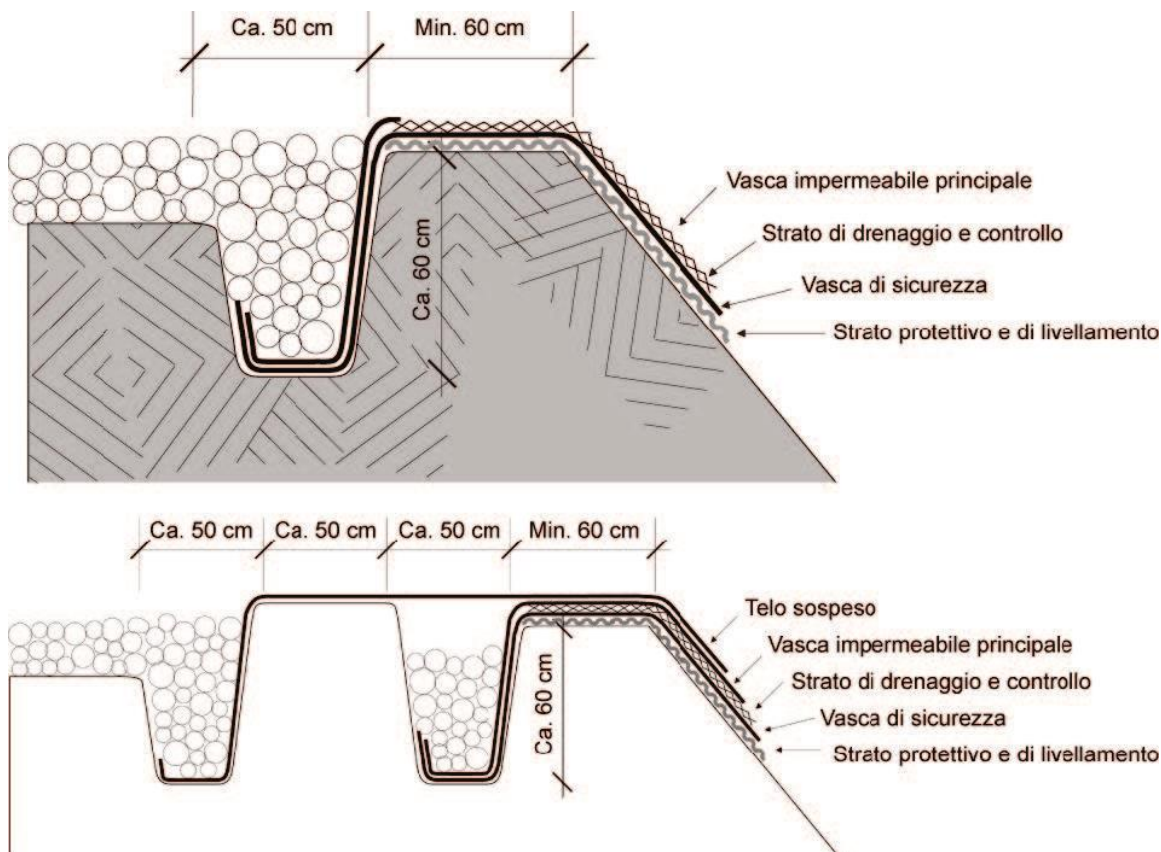
Fig. 17: Trincea di ancoraggio (esempi)
