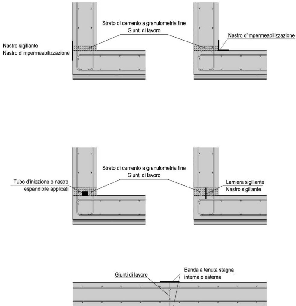
Fig. 2: Serbatoi in calcestruzzo, dettagli esemplificativi di raccordi tra la platea e la parete e per le fasi di betonaggio (platea o parete)
