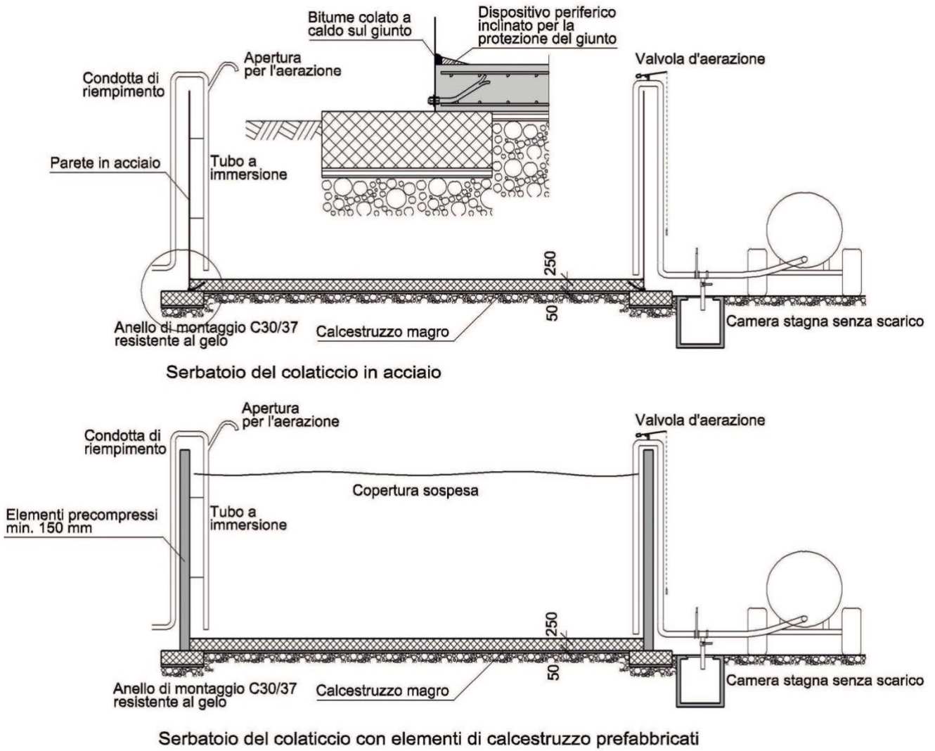
Fig. 7: Esempio di serbatoi posizionati a livello del suolo in acciaio e in elementi di calcestruzzo prefabbricati 63 (dimensioni in mm)
