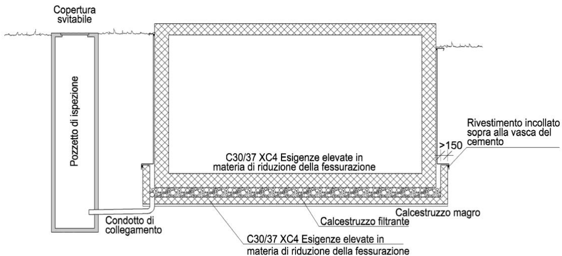
Fig. 14: Esempio di serbatoio del colaticcio con sistema di rilevamento di perdite costituito da vasca in cemento (dimensioni in mm)
